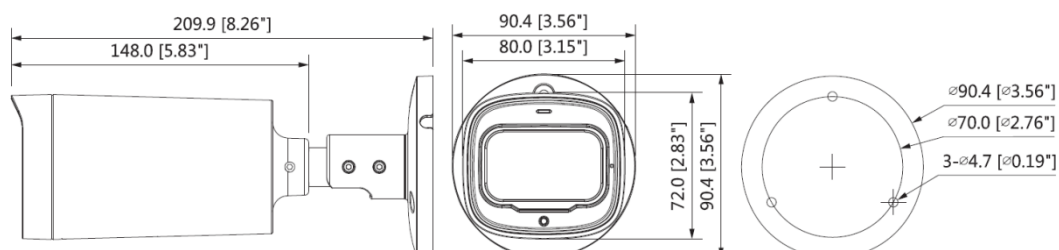
Figure 2-1 (mm [in.])
