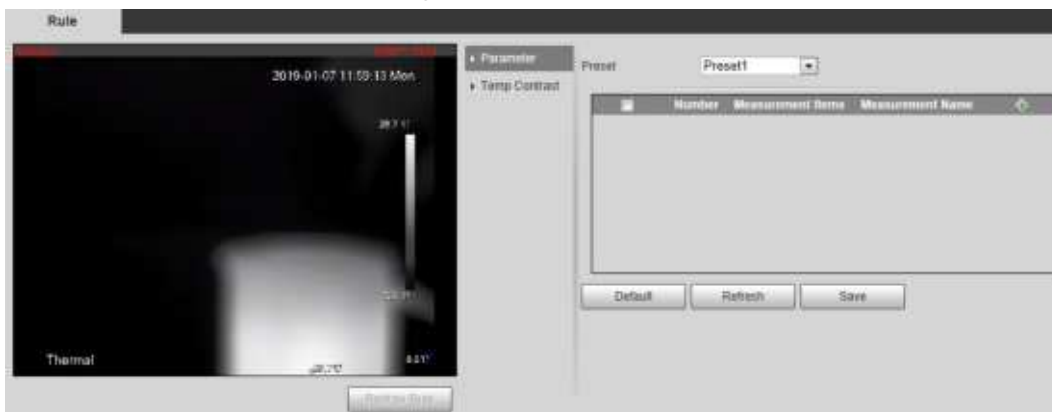
Figure 4-64 Parameter
