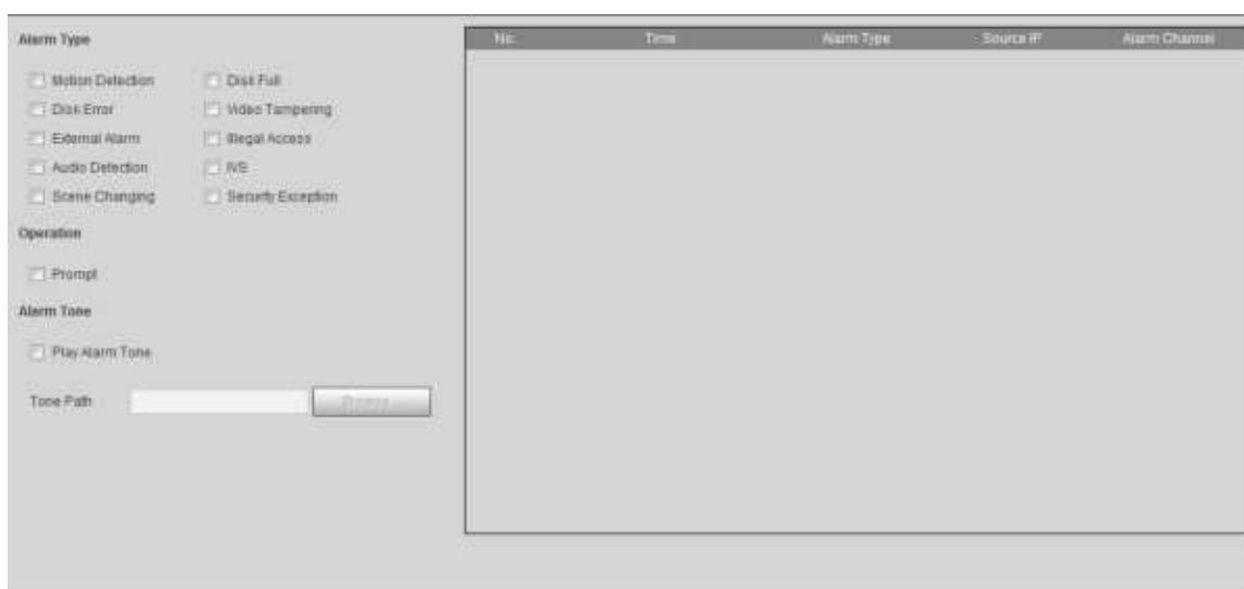
Figure 5-15 Alarm (subscription)
