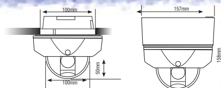
Mini PTZ Dimension
